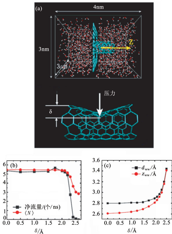
图2 (a)通过向内压碳管上的一个原子来减小通过碳管内水流的方法示意图;(b)通过碳管内净流量(flux)和碳管内水分子的平均个数 \langle N \rangle 与被压碳原子向内移动量 \delta 的关系;(c)被压碳原子两边水分子的距离 d_{ww} 和这个距离沿碳管轴的投影 z_{ww} 随 \delta 的变化
