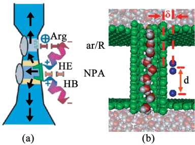
图 3 (a) 影响生物水通道内水流的主要电荷和部分电荷在 ar/R 区域和 NPA 区域(见文献[2]); (b) 模拟系统的组成(绿色小球代表碳原子, 红色小球和白色小球分别代表水分子中的氧原子和氢原子, 蓝色小球代表正电荷, 灰色小球代表负电荷. 模拟系统中包括扶手椅型单壁碳纳米管, 长为 23\text{\AA} , 直径为 8.1\text{\AA} . 3 个电荷的电量分别为 1.0e, 0.5e, 0.5e , 放置在 z = -7.9\text{\AA} , -0.7\text{\AA} 和 0.7\text{\AA} 的位置上, z = 0 代表纳米碳管的中部位置)
