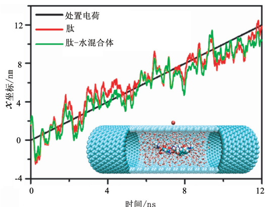
图5 外置电荷对纳米管内水和短肽分子(GNNQQNY)混合体位置的操控(图中直线表示外置电荷的 x 坐标(沿纳米管方向)随时间的变化;曲线表示短肽分子质心的 x 坐标随时间的变化;虚线表示短肽—水混合体质心的 x 坐标随时间的变化.蓝色管状物是碳纳米管的侧视图(为了清晰,部分碳原子在图中未作显示),纳米管正中的链状物为短肽分子(GNNQQNY),短肽分子被水分子(红色小球和白色小球分别代表水分子中的氧原子和氢原子)所包裹.纳米管外的红色圆点为电量 0.5e 的外置电荷)
